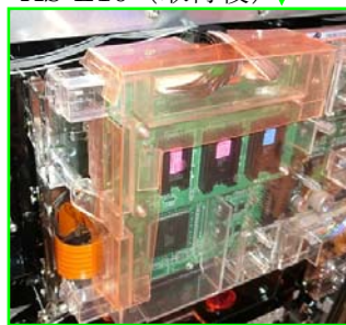
AS-E10（取付後）
