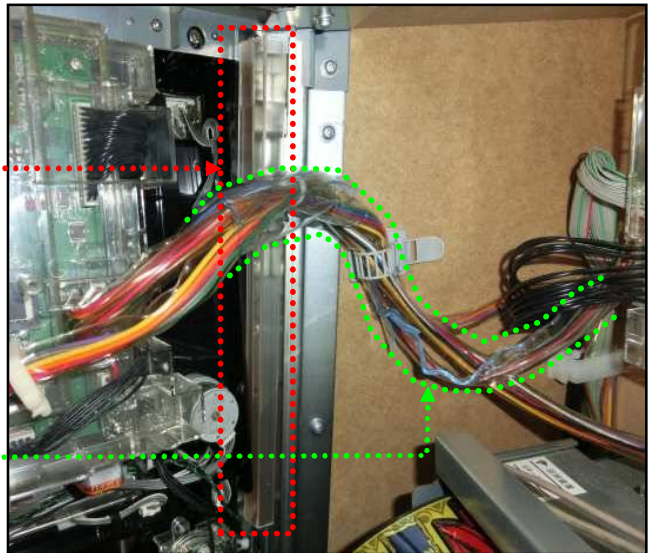
AS-E15、HG-1 対策後
