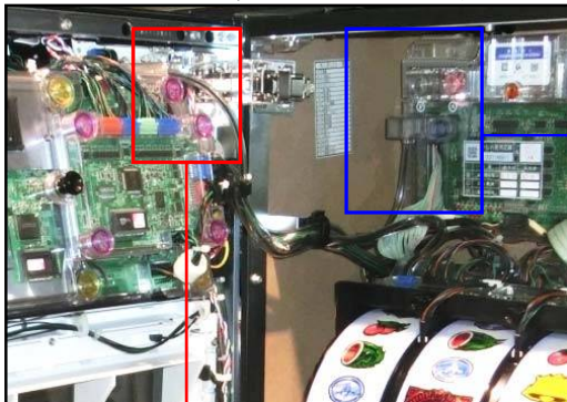
メイン-サブ基板通信ライン全体
